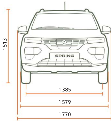
VUE AVANT
