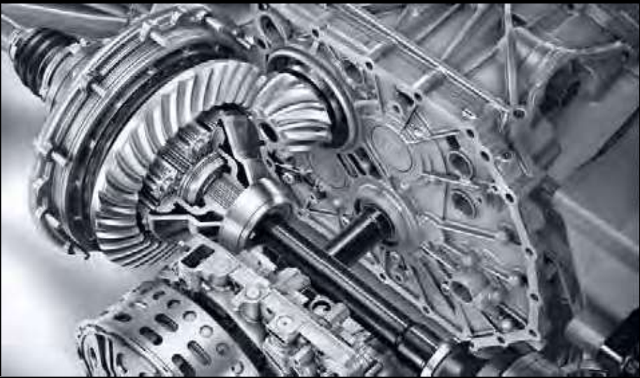
467 - Différentiel électronique autobloquant AMG sur l'essieu arrière
