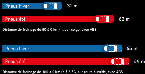
▲ Schéma distance de freinage
